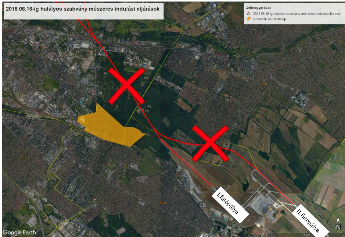
2. ábra 2018. 08.16-ig hatályos szabvány műszeres indulási eljárás (SID)
