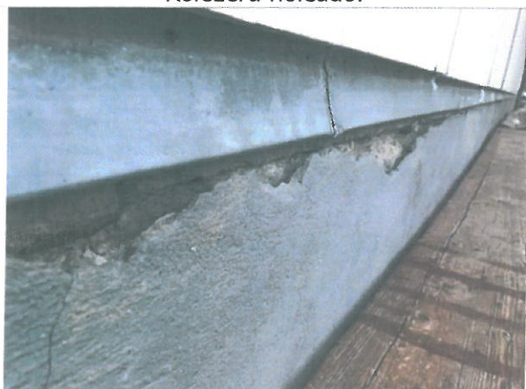
Épülethiba, lábazat.
